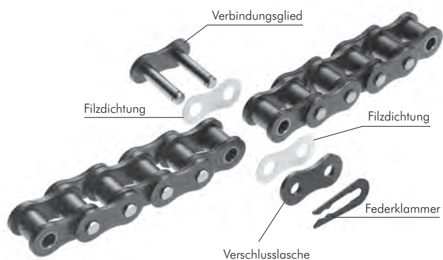
Abb. 12 BS X-LAMBDA Montageverfahren
